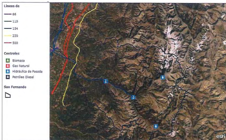
Mapa N°32: Infraestructura Energética San Fernando
